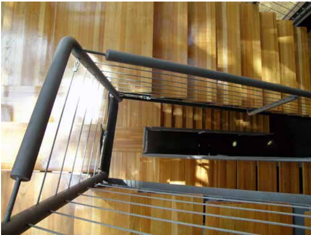
Pasarela. Detalle constructivo de la huella, la baranda, etc. de la escalera (Fotos XL internet [Murcia], 2-8-2005).
